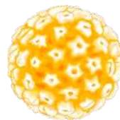
Struktur des Hüllproteins HPV
